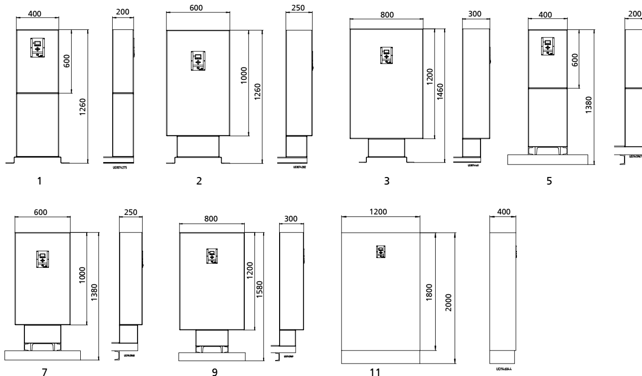
Рис. 4: Габаритные размеры шкафа управления Нуамат К [мм]
