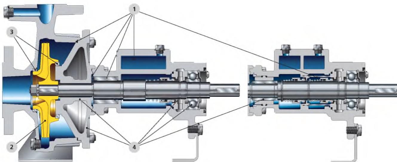
Горизонтальный насос со спиральным корпусом Etanorm SYT с одинарным торцевым уплотнением
