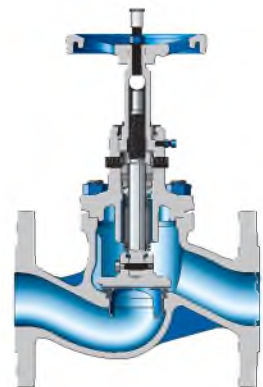
VOA®-H Корончатый конус
